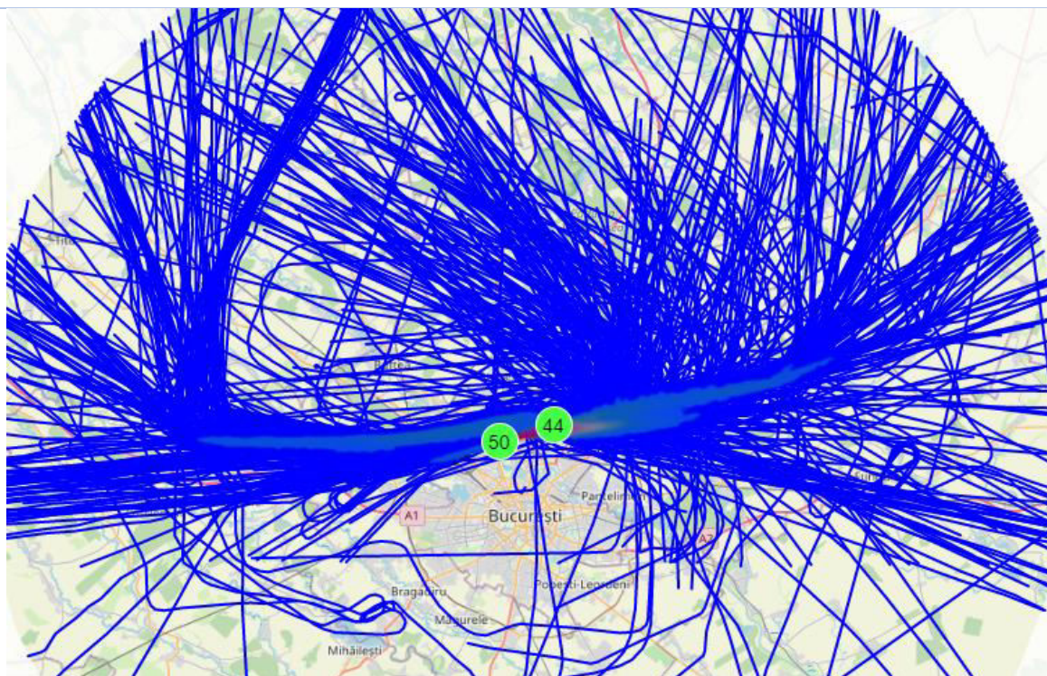
Figura 4.2. (1) - Exemplu de identificare a coridoarelor de zbor decolare pe 07 prin utilizarea densității zborurilor pe \text{km}^2 pana la altitudinea de 5000 m
