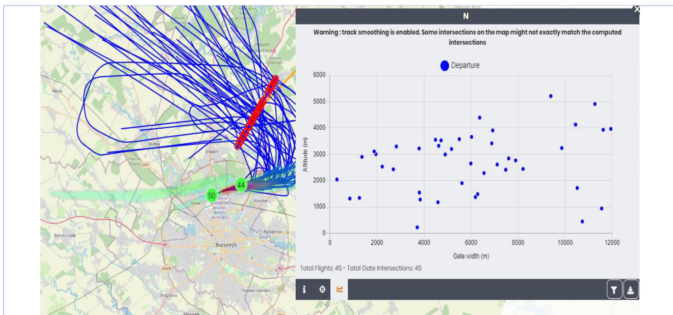
Figura 4.2. (4) - Exemplu de analiza a tipurilor de aeronave care circula pe un culoar de zbor la decolare pe 07
