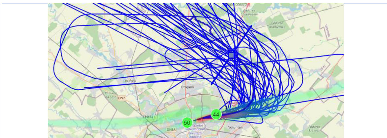
Figura 4.2. (3) - Exemplu de calcul a traiectoriei la sol principale (medii- linia albastra bold) si a dispersiei laterale pe un coridor de zbor identificat pentru decolare pe 07
